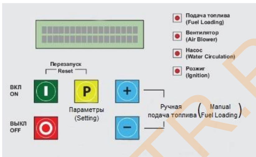
Рисунок 1. Панель управления котла EK3G/S.
