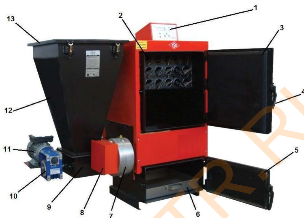
Рисунок 2. Котел EKY/S 50-100 четырехходовая конвективная часть
