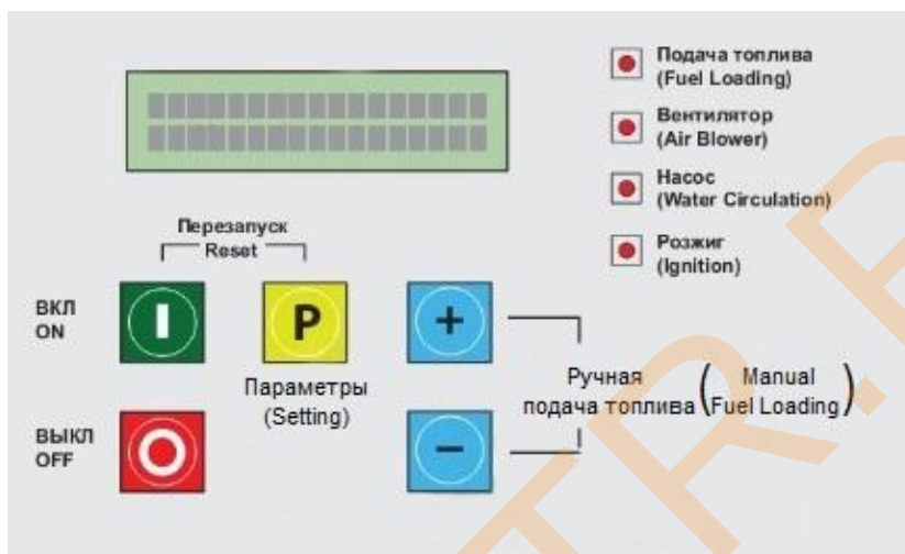
Рисунок 1. Панель управления котла EKY/S.
