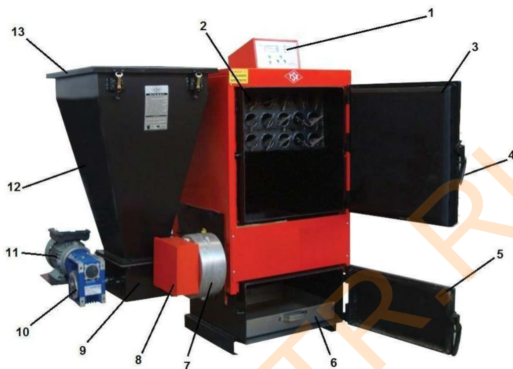
Рисунок 2. Котел ЕKY/S 70-100 четырехходовая конвективная часть
