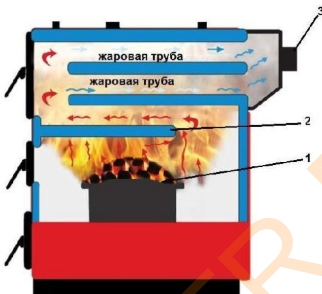
Рисунок 4. Котел EKY/S, схема движения дымовых газов в теплообменнике
